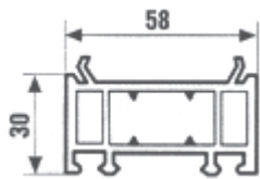
Blendrahmenverbreiterung 3 cm
