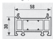
Blendrahmenverbreiterung 3 cm
