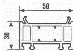
Blendrahmenverbreiterung 3 cm
