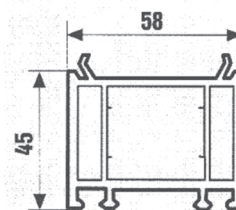
Blendrahmenverbreiterung 4,5 cm
