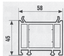
Blendrahmenverbreiterung 4,5 cm
