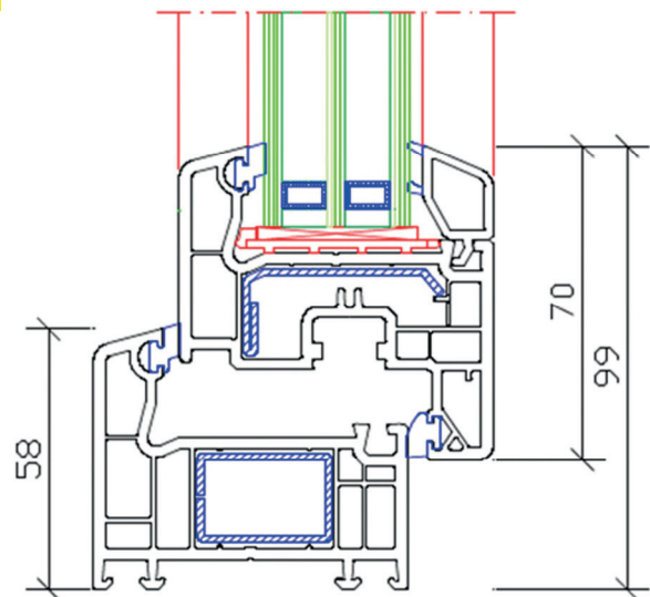
Schnitt ZO DKW Thermo Plus SWISS
