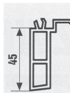
Fensterbankanschlußprofil 4,5 cm
