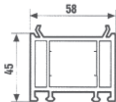
Blendrahmenverbreiterung 4.5 cm
