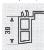
Fensterbankanschlußprofil 3 cm
